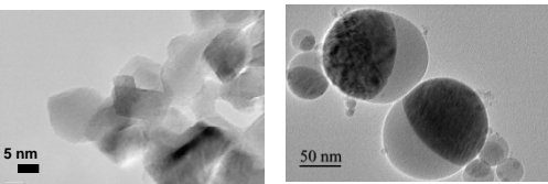
CuO/CeO 2
